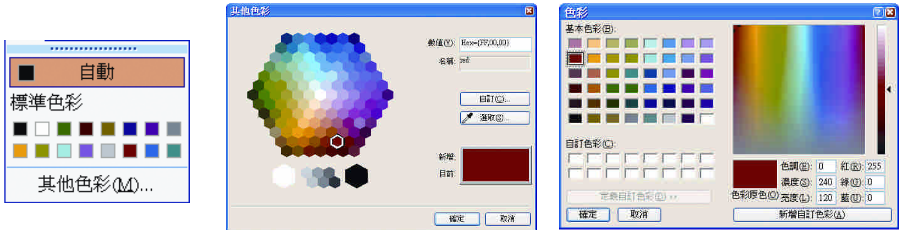
色彩對話框
