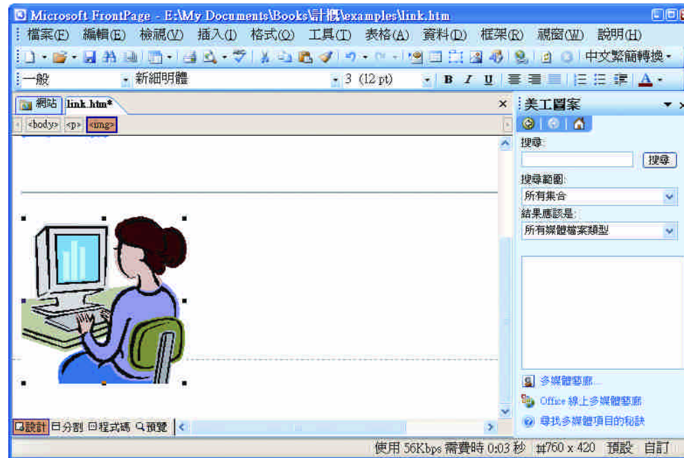
選取圖片
